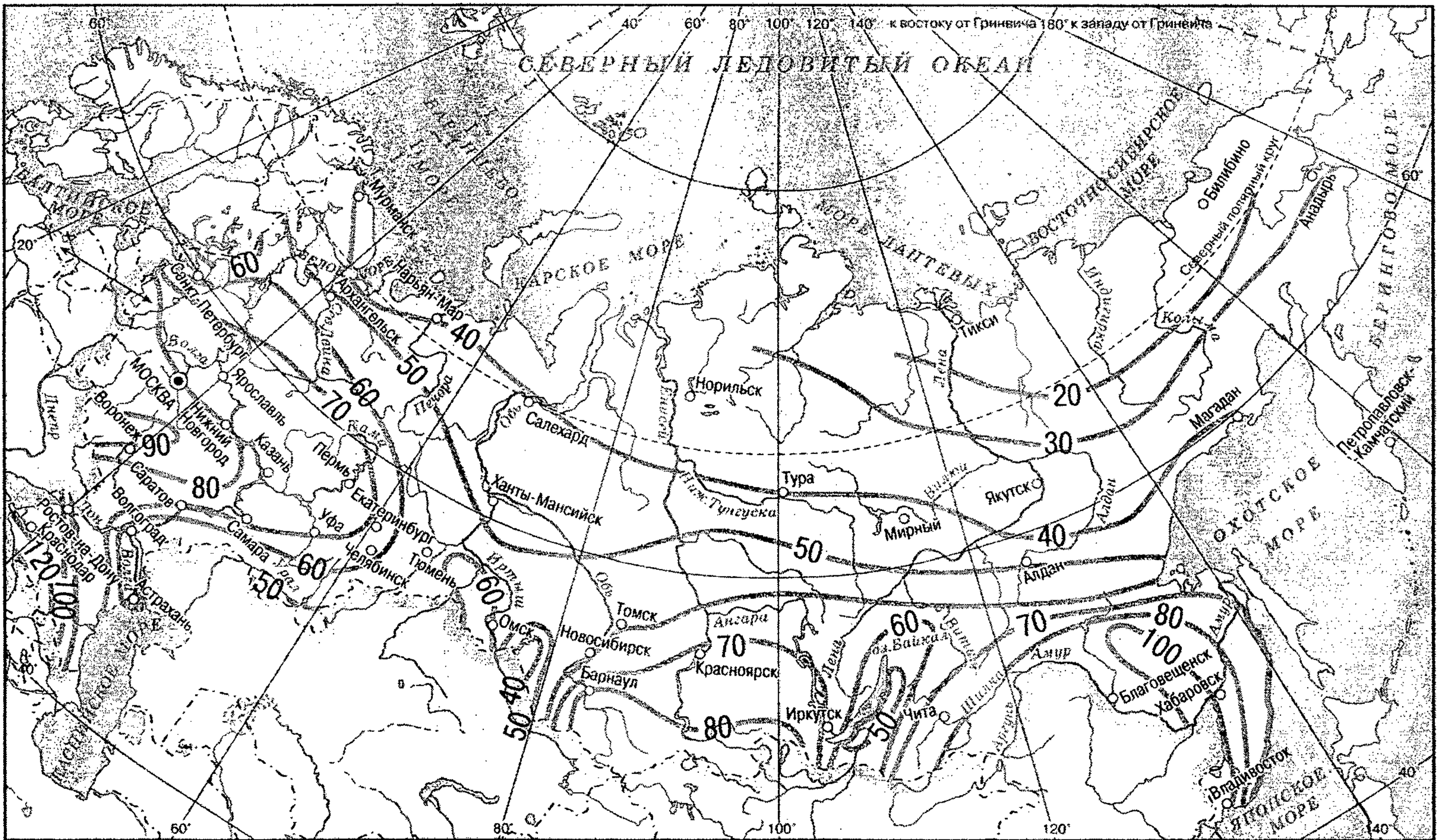
Рисунок Б.1 – Значения величин интенсивности дождя q_{20}
