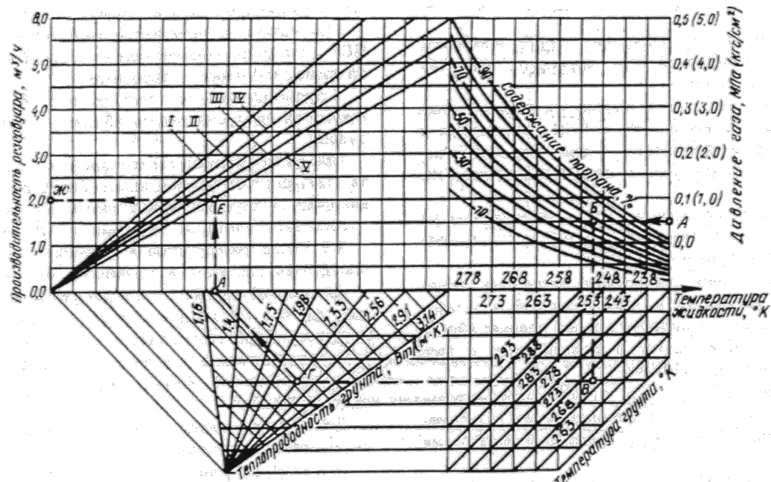
Нограмма для определения производительности резервуара сжиженного газа вместимостью 2,5 и 5 куб.м (подземного)
